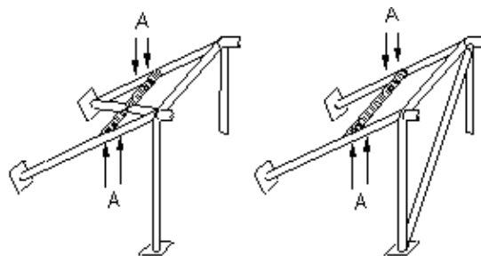
А – отверстия для крепления ремней
